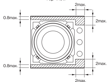
保持・固定可能エリア (斜線部) Top View
