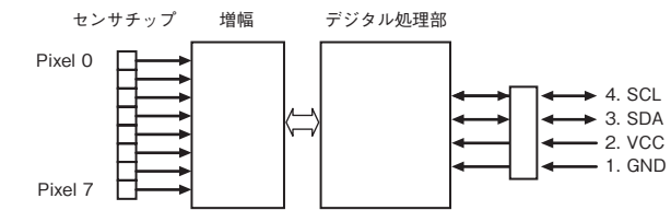
サーマルセンサ構成図 <形D6T-8L-09/09H>
