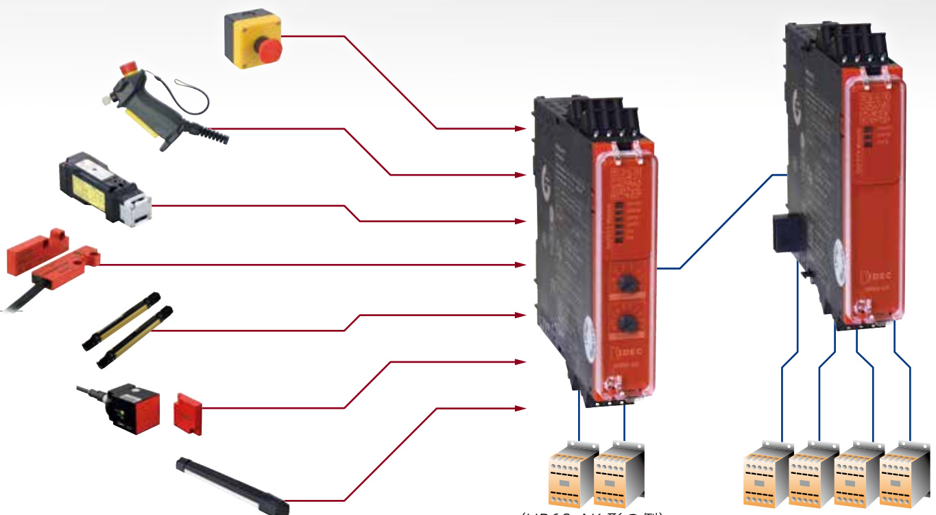
(HR6S-AK 形の例)
