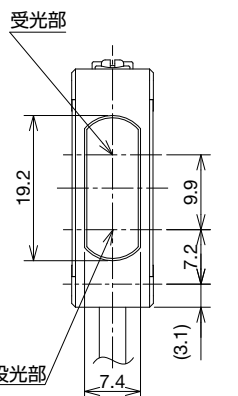
偏光回歸反射形 (SA2E-P)
