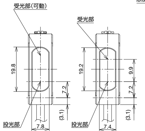
距離設定反射形 (SA2E-B)
