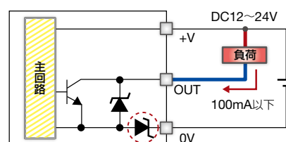
NPN出力 タイプの例
