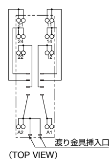
端子配列図
