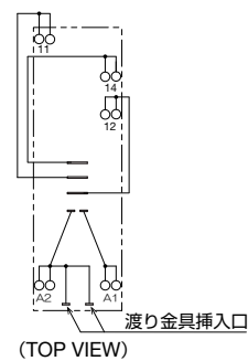
端子配列図
