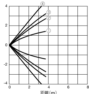
検出体別の検出範囲 (感度レベル：4)
