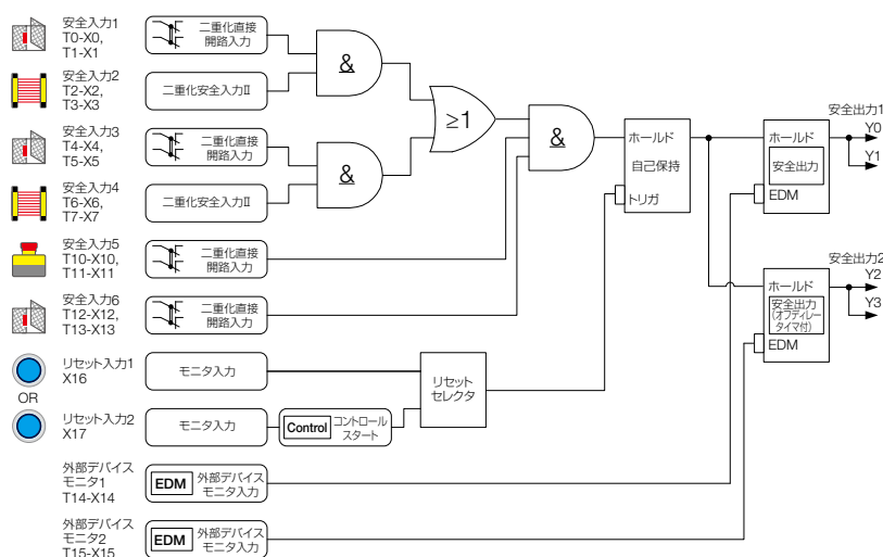
ロジック回路
