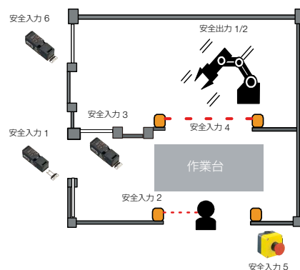
安全システムの構成例
