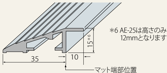
目地枠断面寸法（mm）
