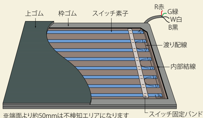
【構造図】
